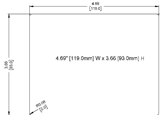
Cutout Dimensions
